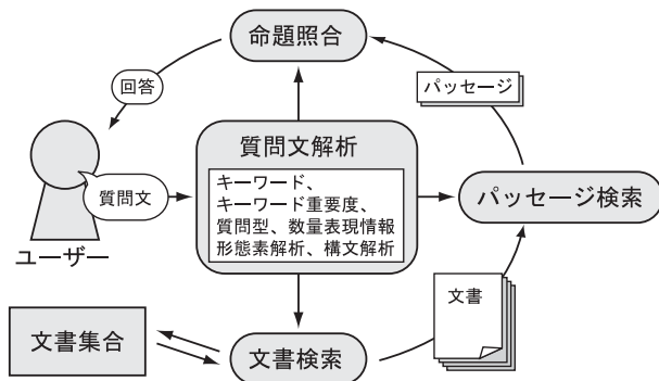
図 1: 質問応答システムの概要
