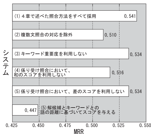
図 2: 照合方法による正解性能の比較
