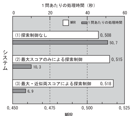
図 3: 探索制御の有無による処理時間と正解性能の比較
